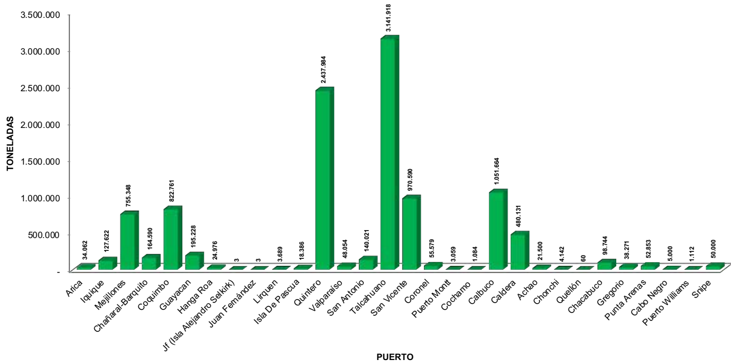
GRÁFICO 17: TONELAJE CARGA LÍQUIDA MOVILIZADO EN CABOTAJE POR PUERTO. AÑO 2023
