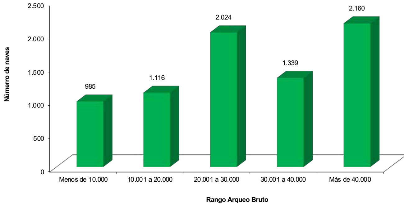
GRÁFICO 9: NÚMERO DE FAENAS DE PRACTICAJE SEGÚN RANGO DE ARQUEO BRUTO. AÑO 2023
