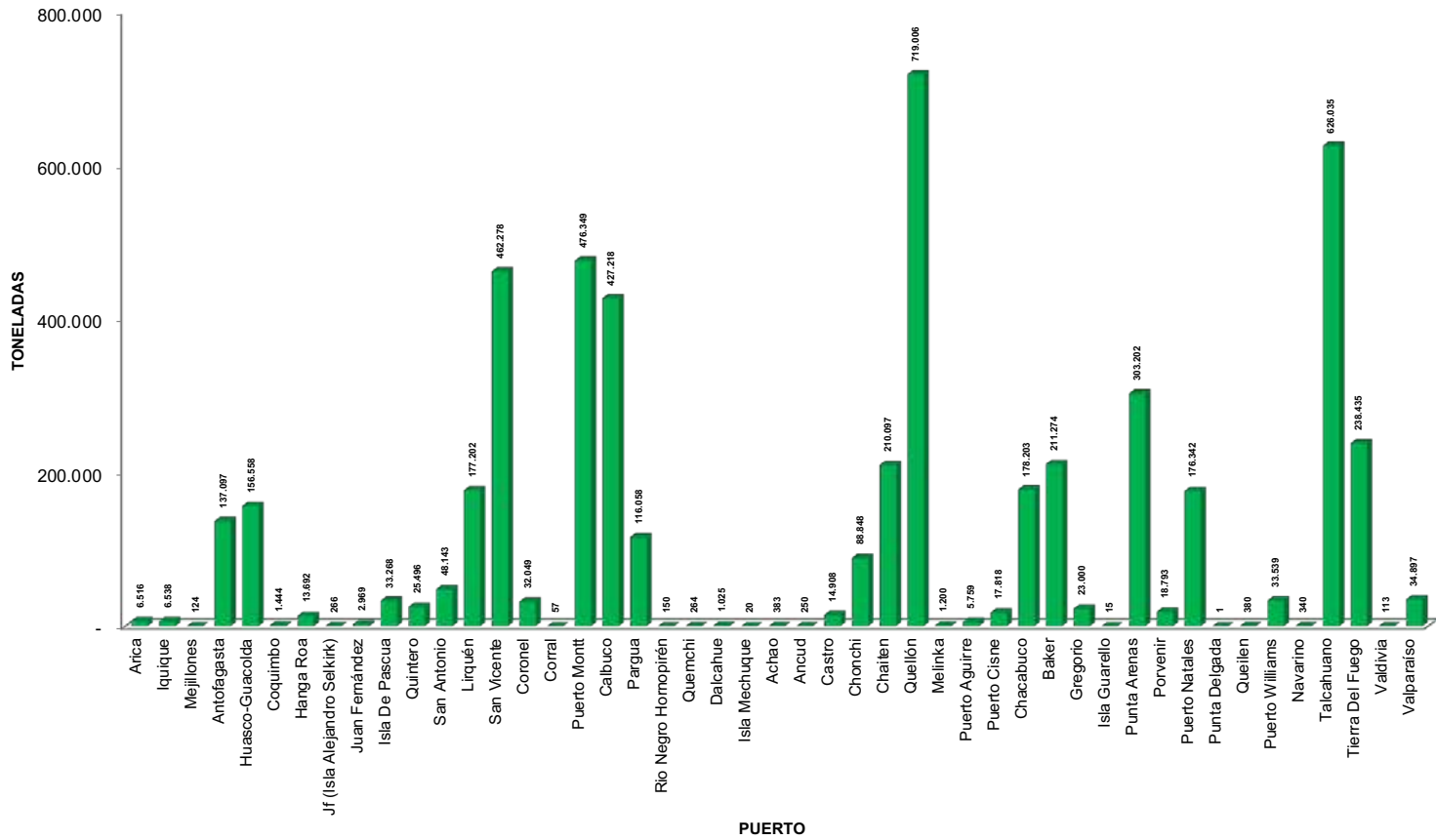
GRÁFICO 15: TONELAJE DE CARGA GENERAL MOVILIZADO EN CABOTAJE POR PUERTO. AÑO 2023
