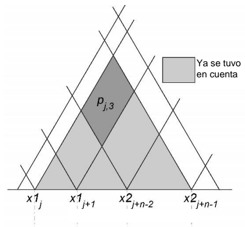
Zonas j j+1 j+n-1 n = 3 : avería en tres zonas
