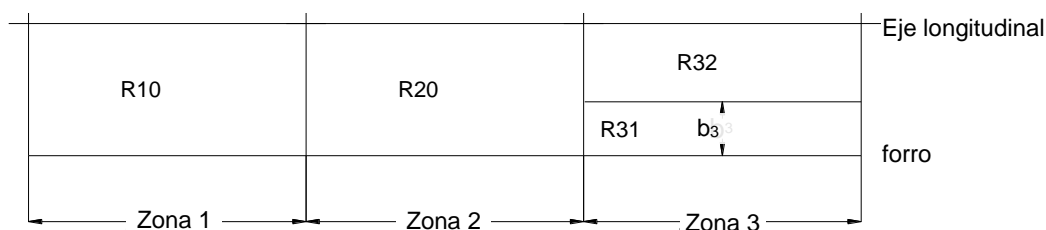
Figura – Las averías combinadas de las zonas 1 + 2 + 3 incluyen una penetración limitada hasta b_3 , teniendo en cuenta la generación de dos averías:
