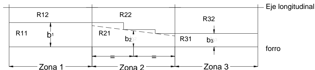
Figura – Avería combinada de las zonas 1 + 2 + 3, incluidas tres penetraciones limitadas diferentes que generan cuatro averías:
