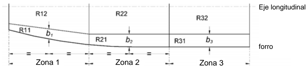
Figura – Avería combinada de las zonas 1 + 2 + 3, incluidas dos penetraciones limitadas diferentes ( b_1 < b_2 = b_3 ) que generan tres averías:
