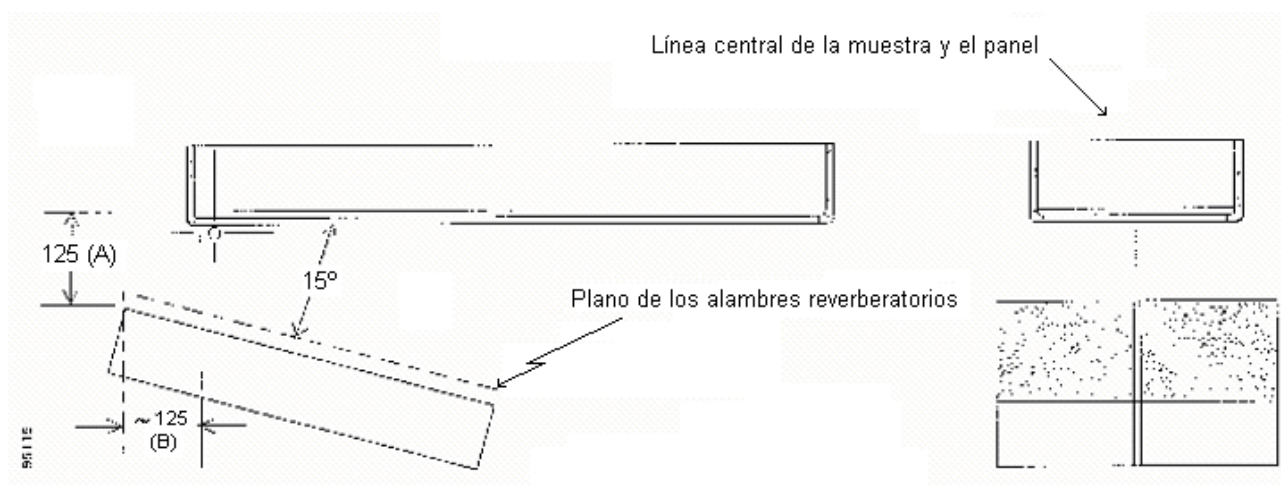
Figura 3 – Disposición de la muestra y el panel
