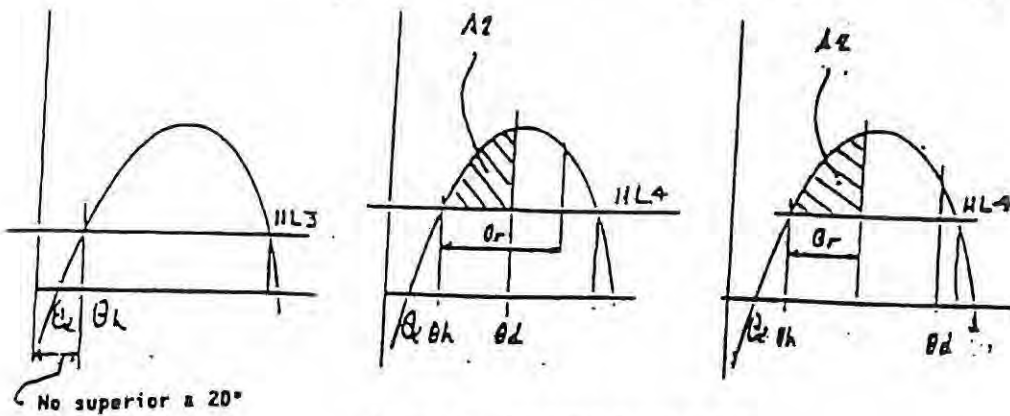
Figura 2 - Estabilidad con avería
