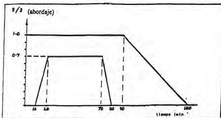
Figura - Envolvente cronológica de la aceleración
