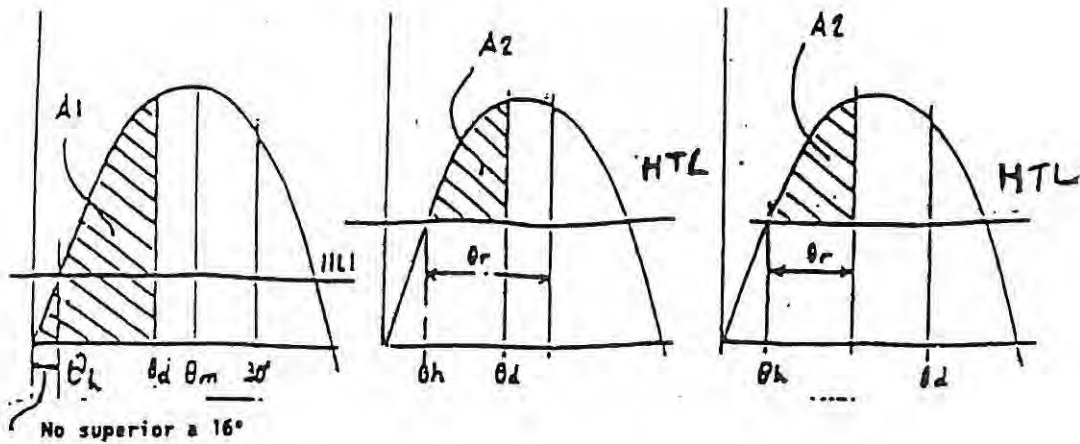
Figura 1 - Estabilidad sin avería
