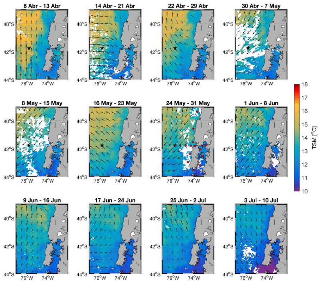
Figura 21b. Campos semanales de Temperatura Superficial del Mar (MODIS-Aqua, 1 km de resolución espacial) y viento satelital (ASCAT, 25 km de resolución espacial) en el mar interior y zona oceánica frente a Chiloé entre abril y julio 2016. El vector vertical ubicado sobre tierra indica la escala de los vectores de viento, y corresponde a una velocidad de 20 km h -1 . El símbolo negro con forma de estrella indica el punto de vertimiento de salmones en marzo 2016. Los puntos rojos en el panel de 24-31 mayo indican la posición de las estaciones de muestreo visitadas durante el crucero a bordo del Cabo de Hornos. Datos MODIS-Aqua fueron procesados y proporcionados por G. Saldías (Oregon State University, USA).
