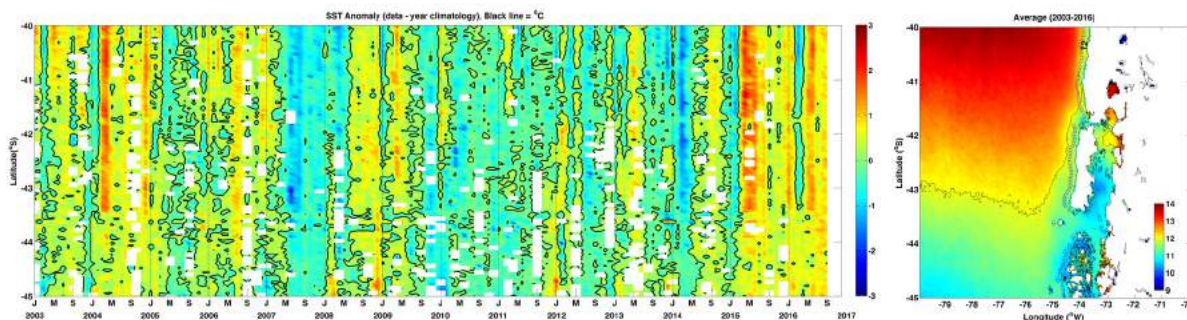
Figura 24. Anomalías diarias de la Temperatura Superficial del Mar (°C) detectada por MODIS-Aqua entre 2003 y 2016 para pixeles cercanos a la costa entre 40 y 45 °S. Los tonos amarillos-rojos y verdes-azules muestran condiciones más cálidas y más frías que lo normal, respectivamente. Los contornos negros indican diferencia cero. El mapa de la derecha muestra la ubicación de los pixeles utilizados en este análisis. Figura gentileza de D. Narváez (U. de Concepción).
