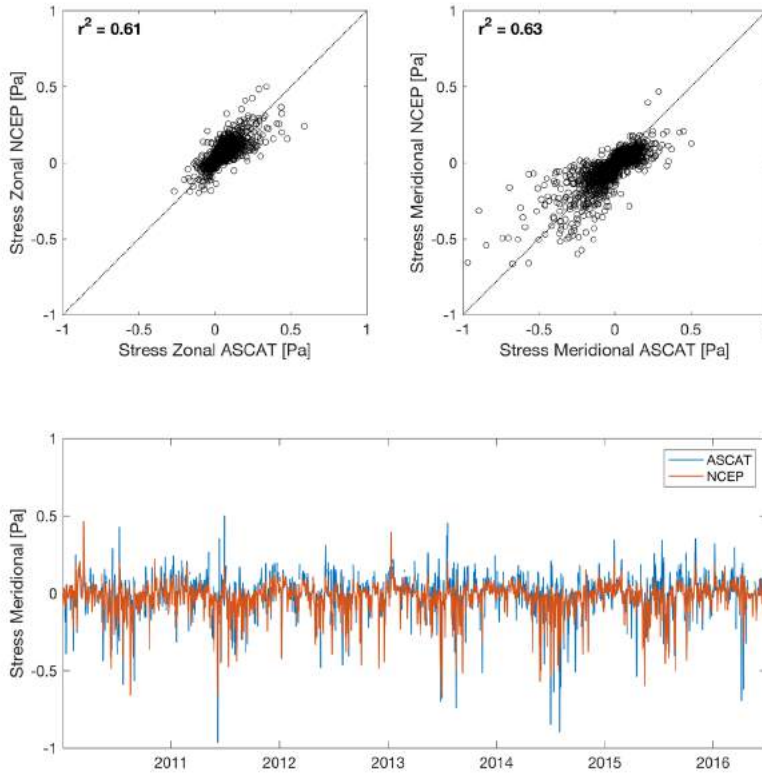
Figura 18. Comparación del stress de viento estimado a partir de imágenes satelitales ASCAT y el estimado por re-análisis. Los paneles inferiores muestran la correlación entre los componentes zonal y meridional del viento para ambas fuentes de información. El panel inferior muestra la correspondencia en fluctuaciones diarias del componente meridional del viento para el periodo 2009-2016.
