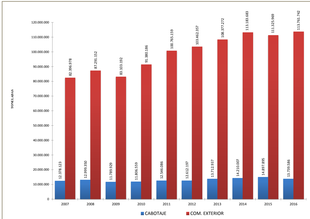
Gráfico 10: Tonelaje movilizado por servicio. Años 2007 - 2016
