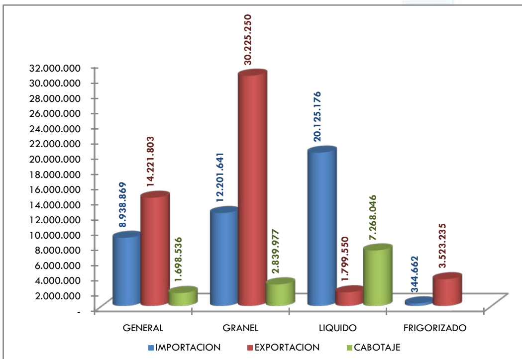
Gráfico 11: Tonelaje movilizado por tipo de carga. Año 2010
