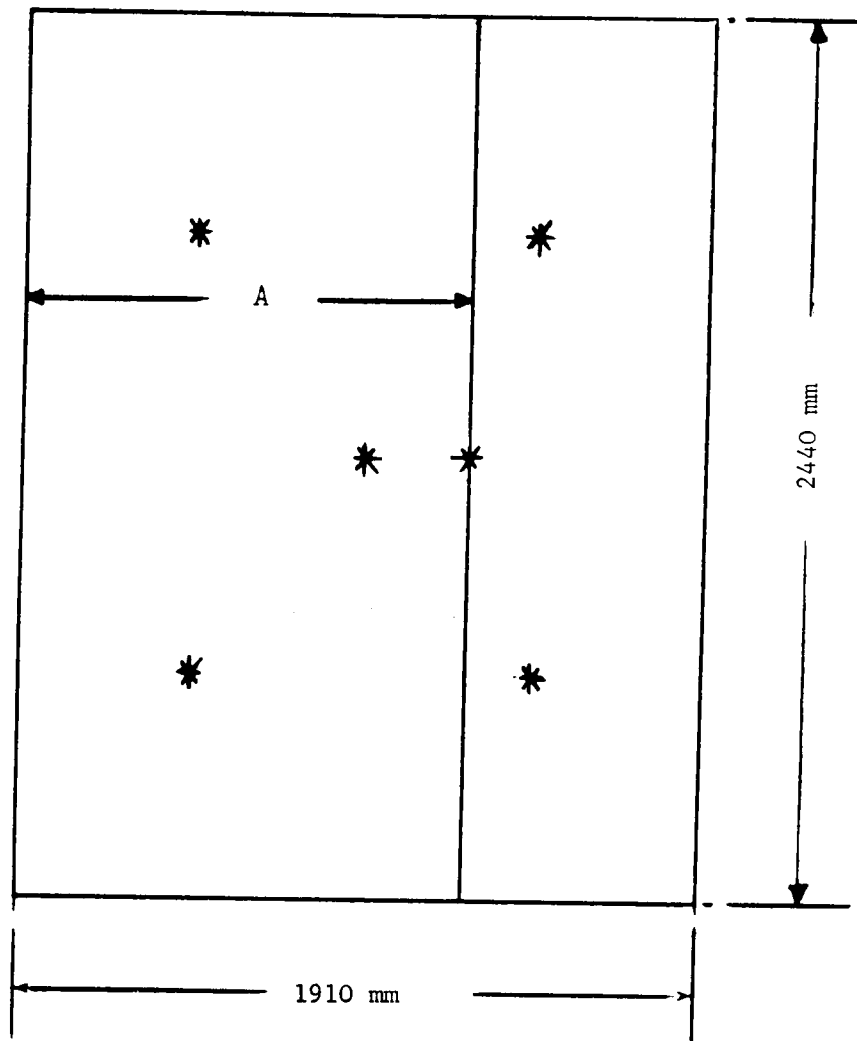
ELEVATION
